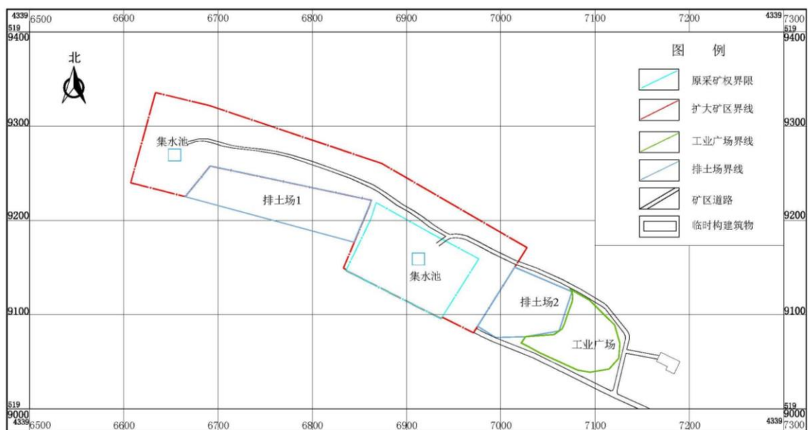
图 1-3 矿山平面布置图
