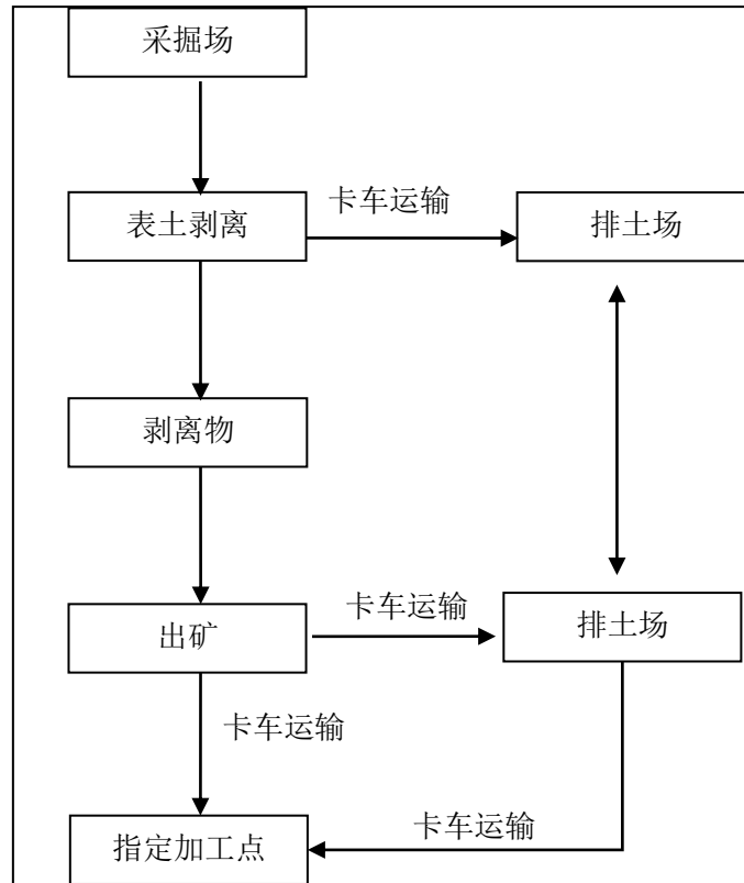
图 3-1 项目生产工艺流程及土地损毁流程图
